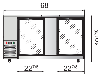
MBB69G-GR
